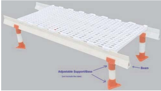
雞用地板 (120x50x4cm;2kg/pcs)
