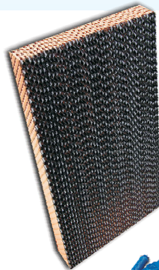
715.002E #7090 水簾帶黑膠 (180*60*15cm) #7090 cooling pad with BC (180*60*15cm)
